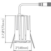
1" MODULE
