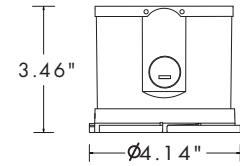
20W IC
